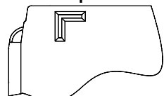
Разрез В-В: уплотняющая кромка EPDM
